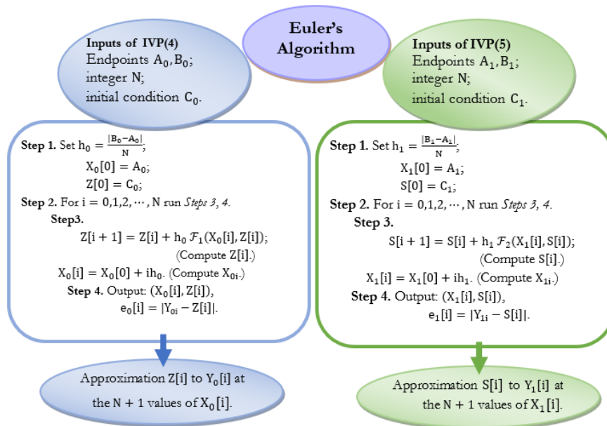
Fig. 1. Euler’s algorithm.
